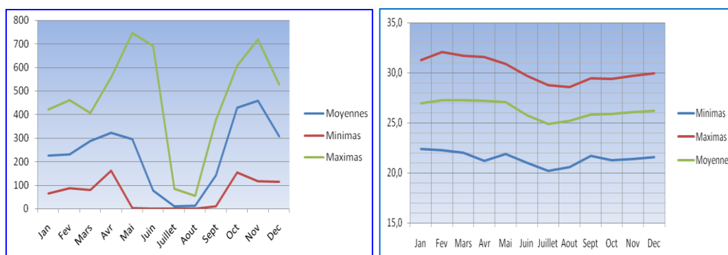
Figure 8 : Répartition des précipitations au Gabon Source : DGEPF, 2013 6
